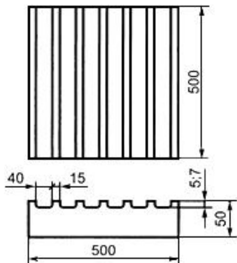
Рисунок 1 - Форма рифления с продольными рифами
