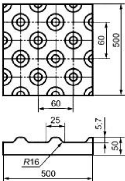
Рисунок 2 - Форма рифления с конусообразными рифами
