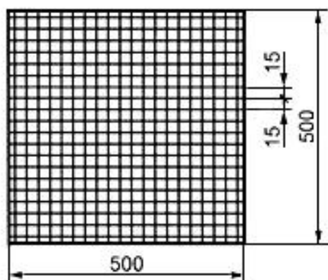
Рисунок 3 - Форма рифления с квадратными рифами
